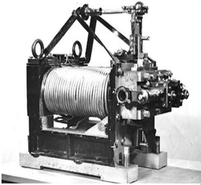
Das von Einthoven entwickelte Saitengalvanometer zur Aufzeichnung von EKGs
